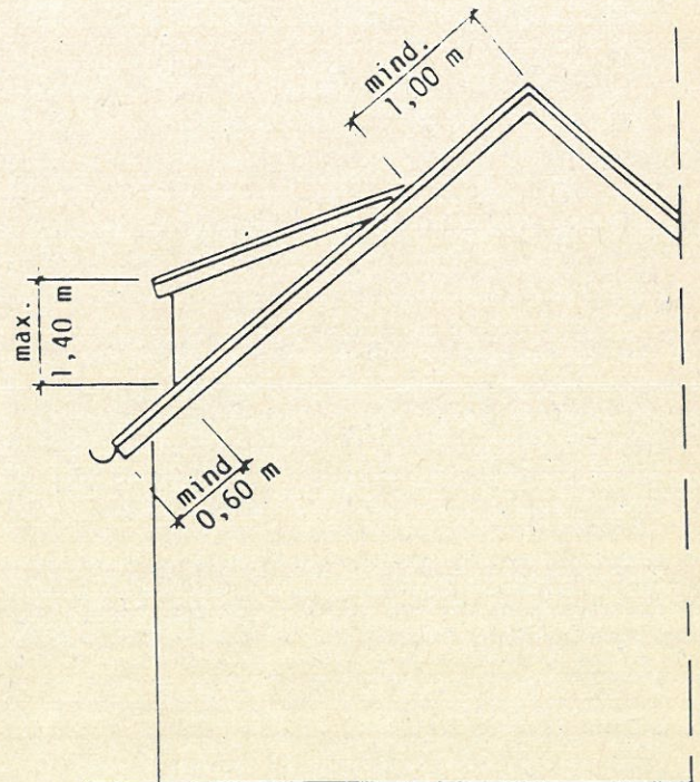
SCHLEPPGAUBE
