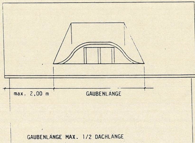
OCHSENAUGENGAUBE
